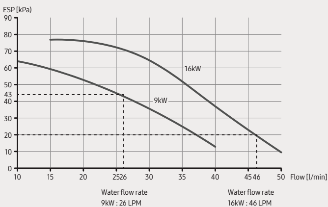
1) Diagramma curve prevalenza portata
