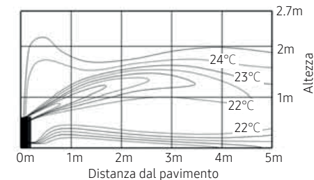
(2) Distribuzione della temperatura [raffreddamento]
