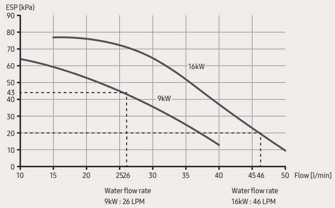
1) Diagramma curve prevalenza portata
