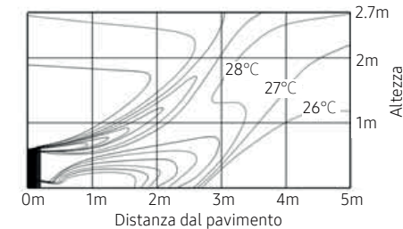
(4) Distribuzione della temperatura dell'aria [riscaldamento]
